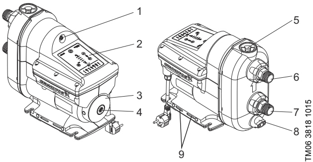
Fig. 10 Grundfos SCALA pump
